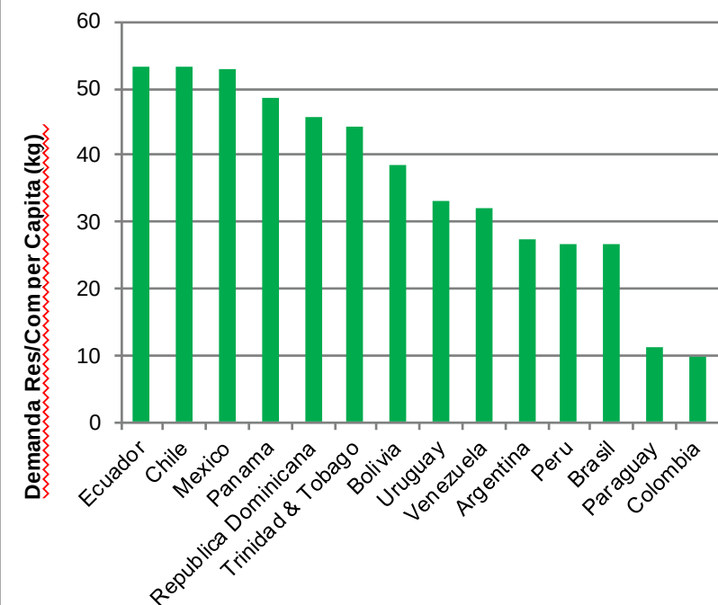
Demanda Residencial y Comercial per capita en America Latina
